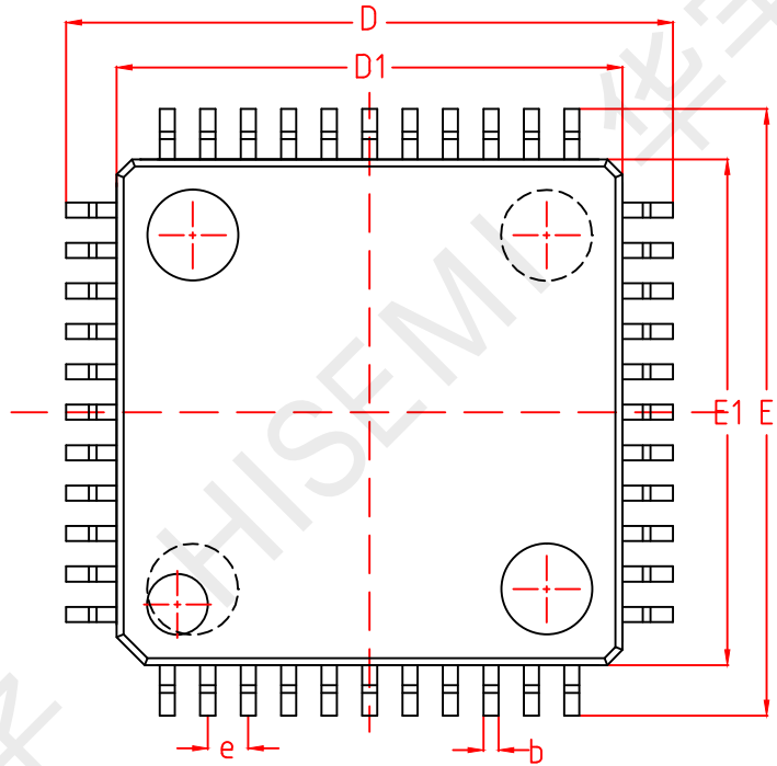
TOP VIEW 正视图
