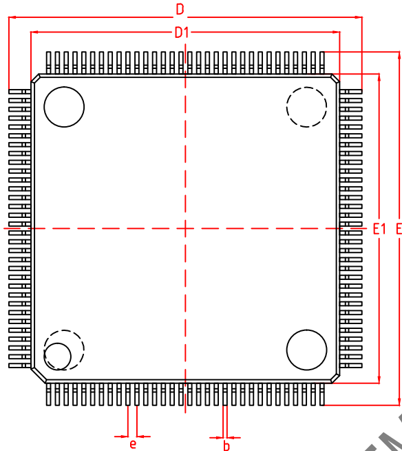
TOP VIEW 正视图
